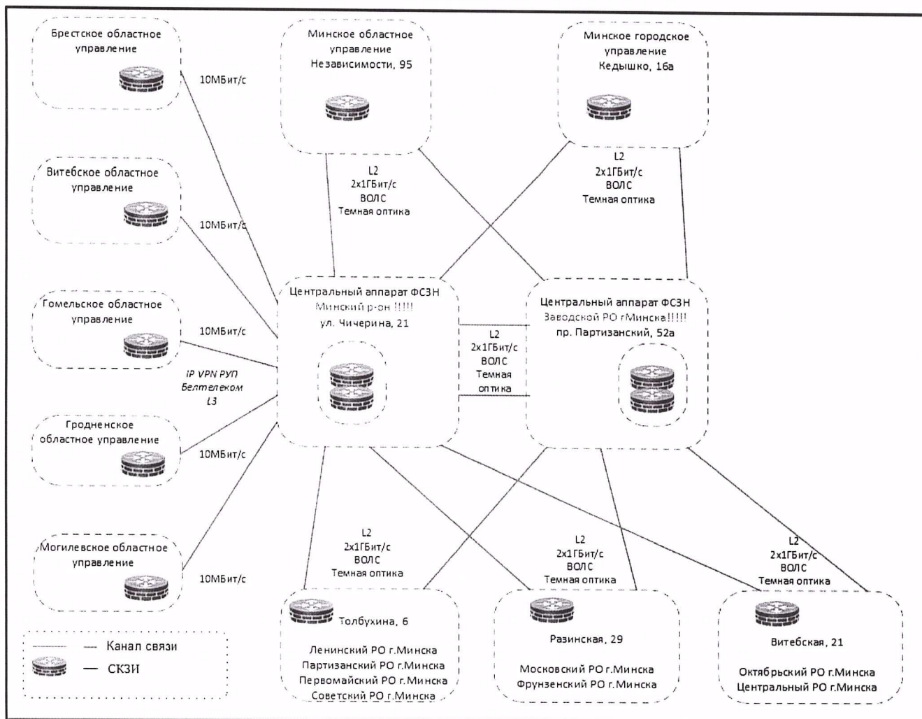
Рис.1. Структурная схема каналов связи в корпоративной сети Фонда
